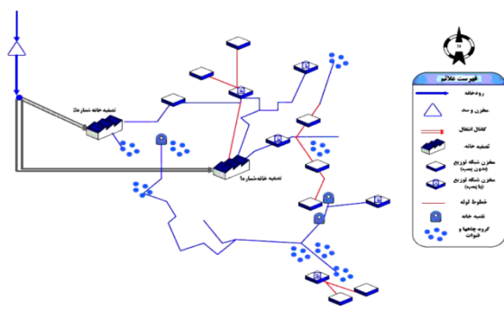
شکل ۸) نمونه سیستم تامین و توزیع آب شهری
